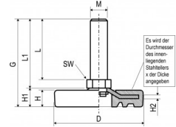
M 8 mit Innensechskant SW4 im Gewindeende
